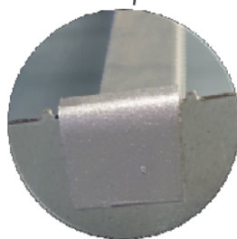
Ergots de centrage pour la pose du support caillebotis
